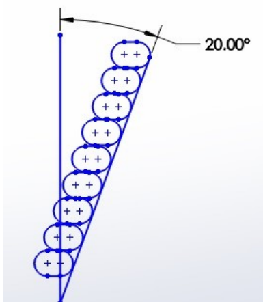
Fig. 25-5: 20 deg. overhang.
