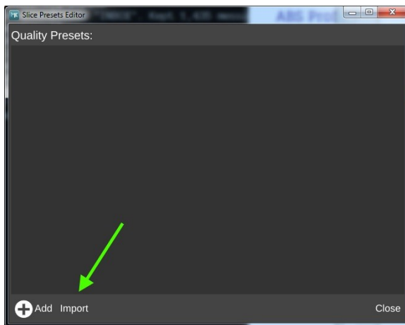
Fig. 20-2: Import!
