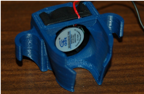
Fig. 20-23: Fan installed, inside view.
