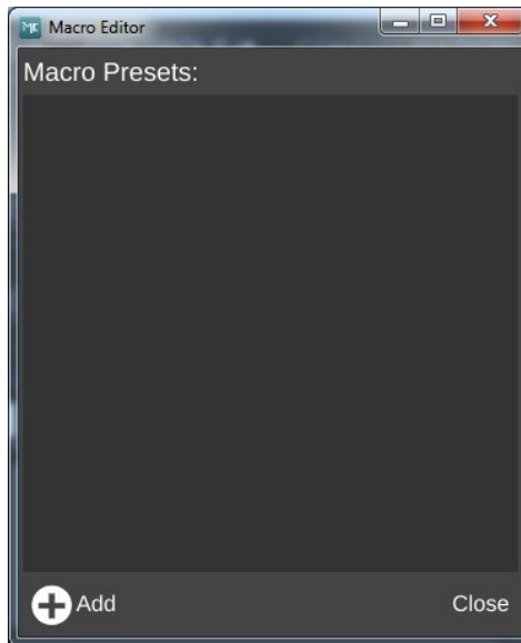
Fig. 19-30: Macro Editor.
